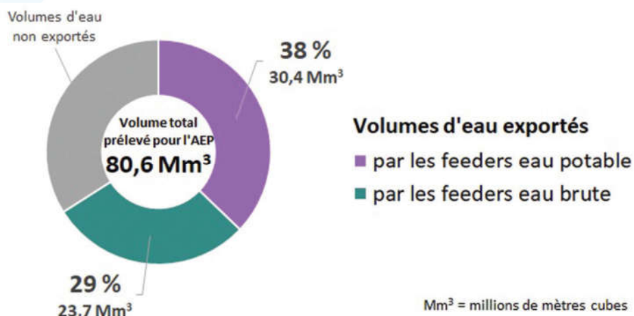
Figure 13 : Volumes exportés pour l'AEP par les grandes infrastructures de transfert d'eau en 2018 (source : Observatoire de l'Eau)
