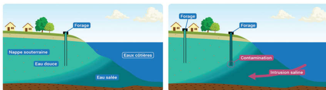
Figure 5 : Représentation du phénomène d'intrusion saline (source : Eaufrance)
