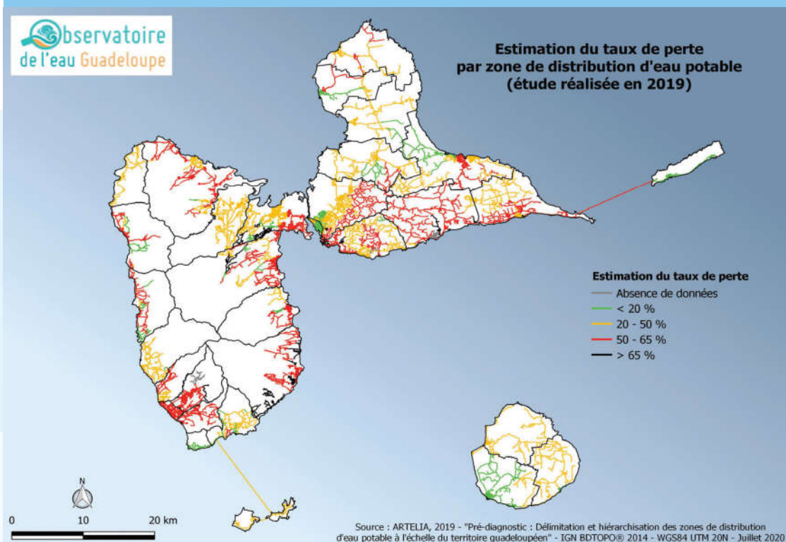
Figure 23 : Estimation du taux de perte par zone de distribution d'eau potable (source : ARTELIA, 2019)
