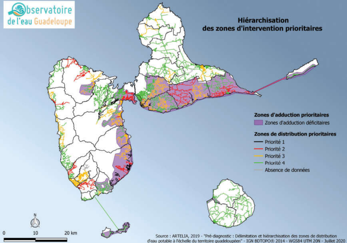
Figure 46 : Hierarchisation des zones d'intervention prioritaires (source : ARTELIA, 2019)
